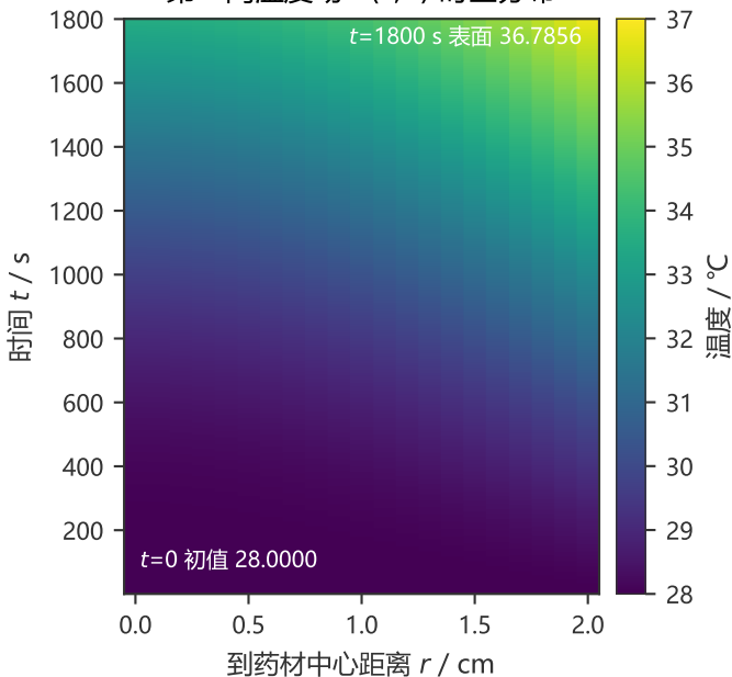
第一问温度场 T(r, t) 时空分布
