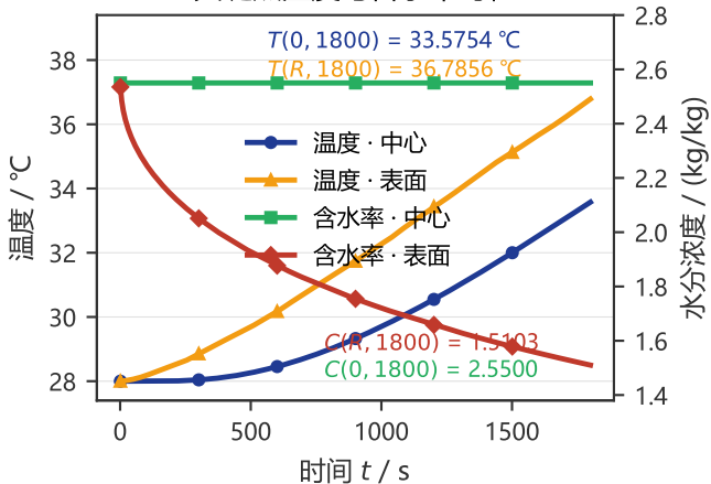
关键点温度与含水率时程
