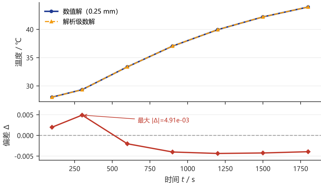
温度解析对拍 (常边界特例, r = 0 )
