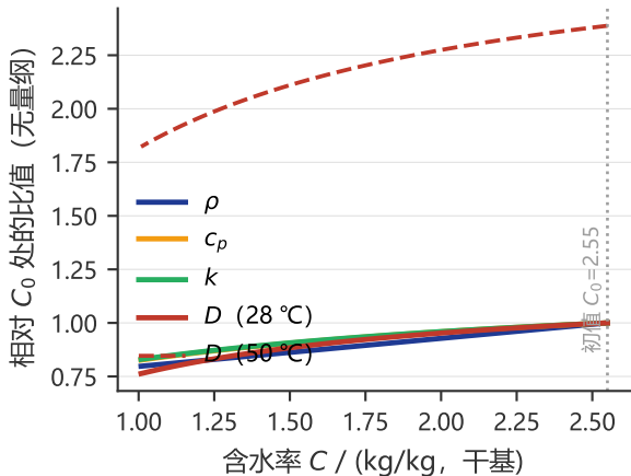
第二问物性随含水率的演化
