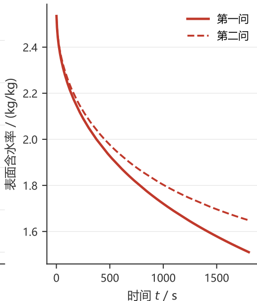
(b) 表面含水率
