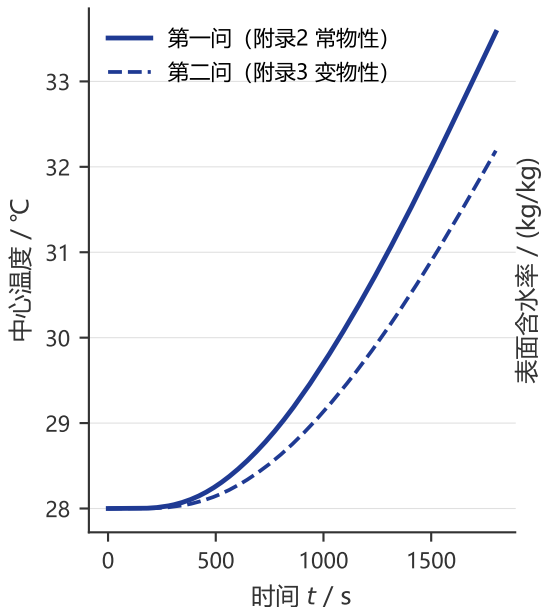
(a) 中心温度
