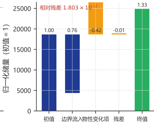
(b) 能量收支 (须含物性变化项)
