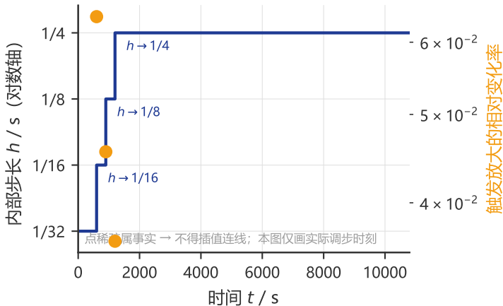
Q2 自适应步长轨迹 (阶梯, 仅 3 个调步点)
