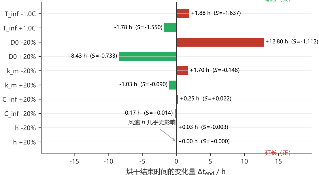
第三问烘干结束时间的参数灵敏度 (基准 57.53 h)
