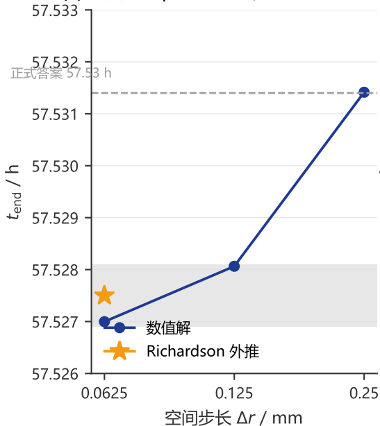
(a) 空间维: p = 1.650 , GCI = 0.0011\% (b) 时间维: 非单调 (不适用 Richardson)
