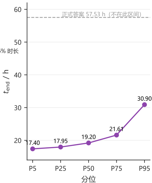
(b) 分位区间（先验 C_{\text{fr}} \sim U[0.15, 1.0] ，主观设定）
