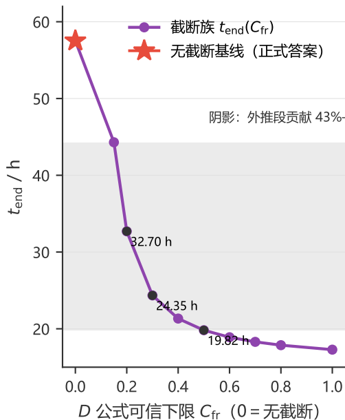
(a) 确定性截断族
