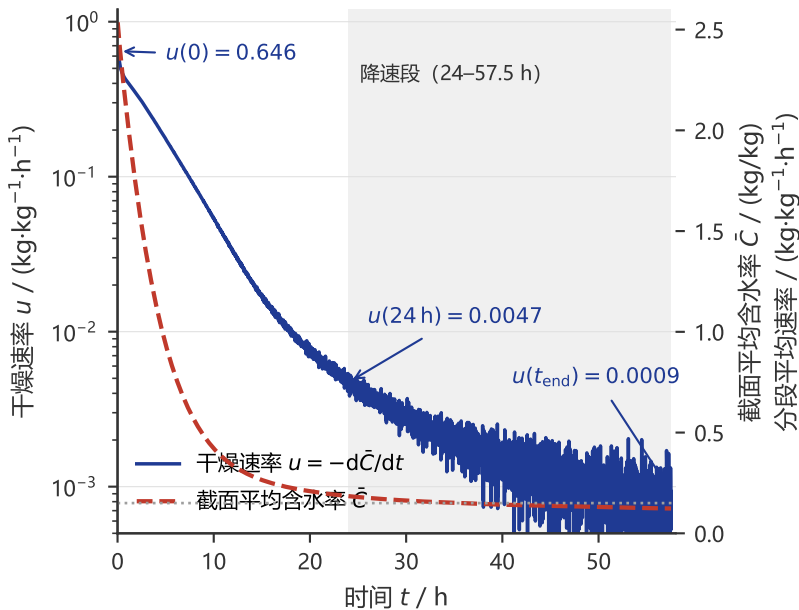
截面平均含水率与干燥速率的时间演化（速率取对数轴）
