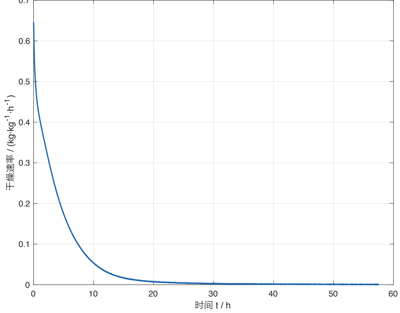
Q3 干燥速率曲线
