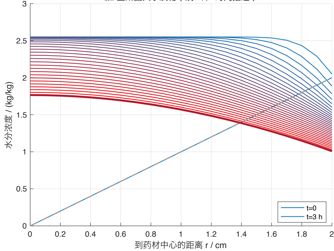
Q2 全断面失水演化 ( 浅->深=时间推进 )
