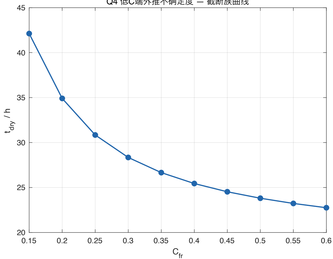
Q4 低C端外推不确定度 — 截断族曲线
