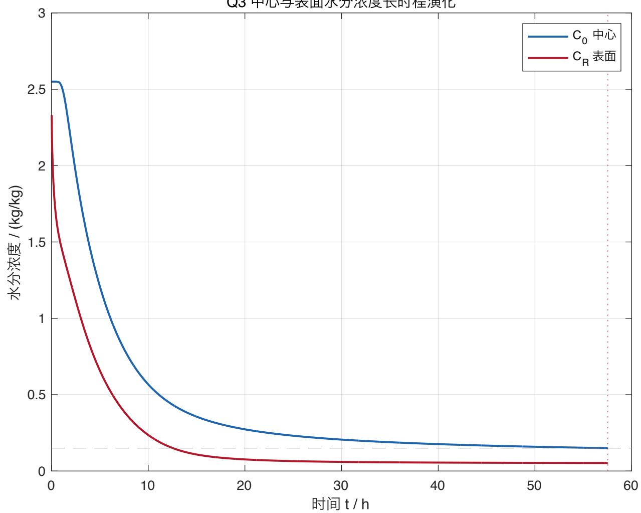
Q3 中心与表面水分浓度长时程演化
