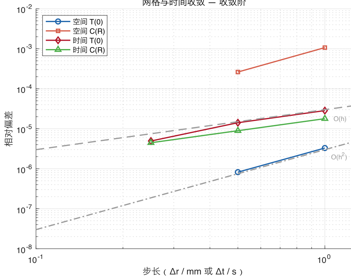
网格与时间收敛 — 收敛阶
