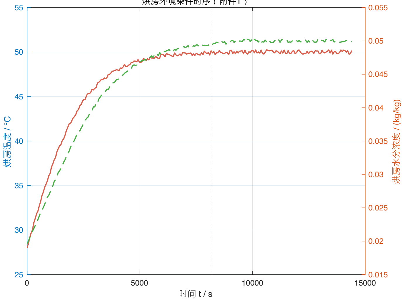
烘房环境条件时序 ( 附件1 )
