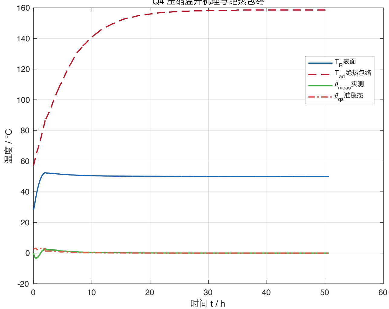
Q4 压缩温升机理与绝热包络
