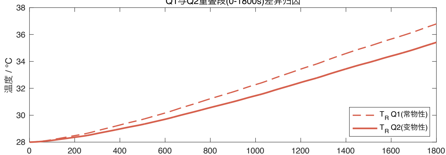
Q1与Q2重叠段(0-1800s)差异归因
