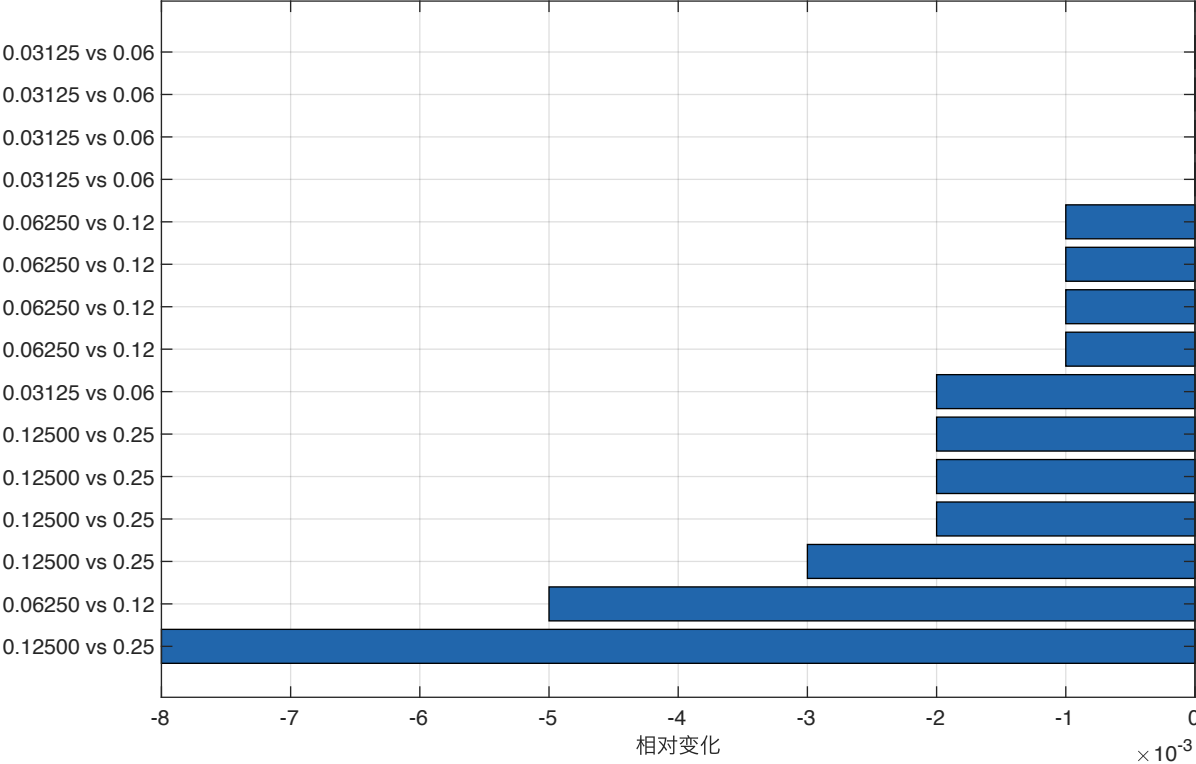
Q3 收敛性 — 各位置收敛情况
