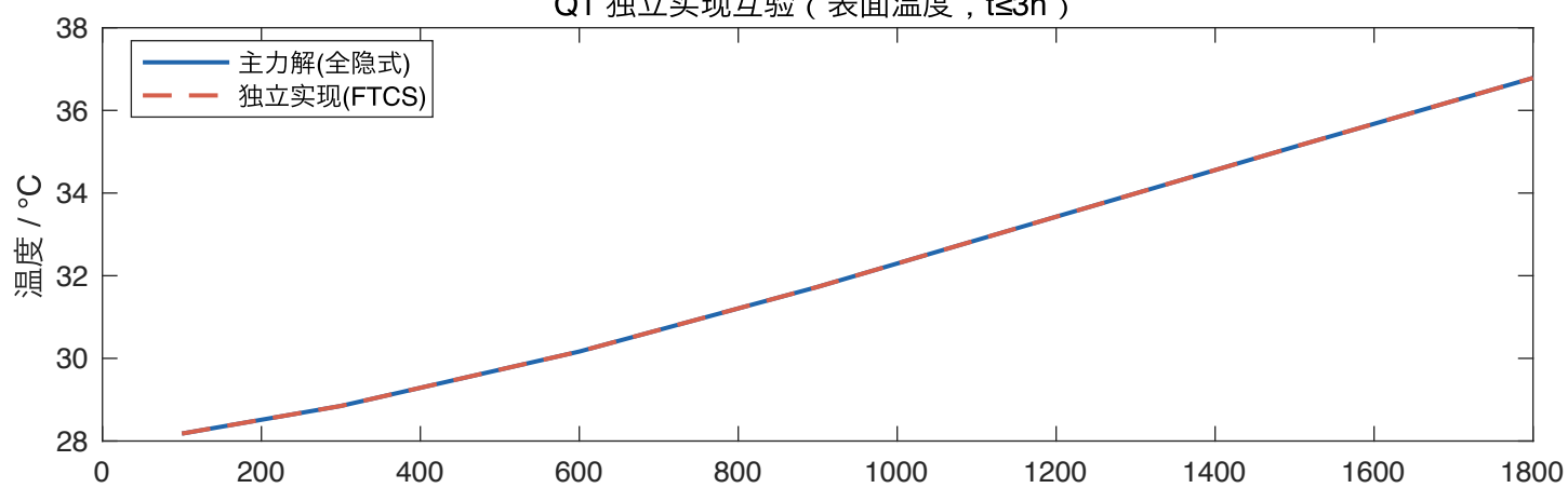
Q1 独立实现互验 ( 表面温度, t \leq 3h )
