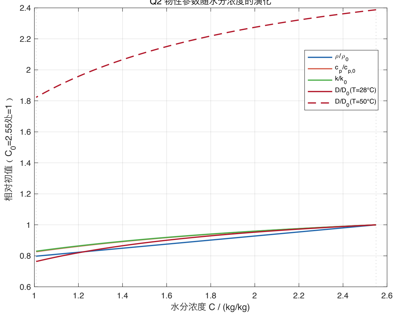
Q2 物性参数随水分浓度的演化
