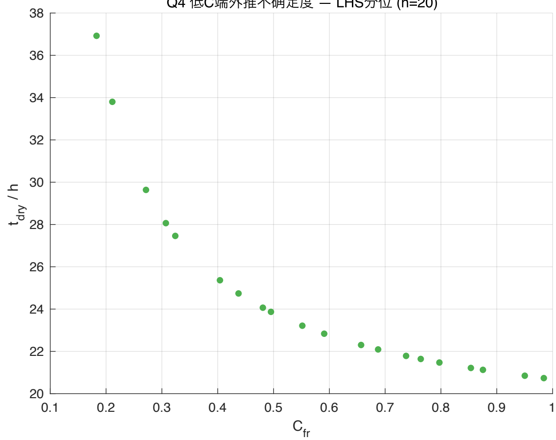
Q4 低C端外推不确定度 — LHS分位 (n=20)
