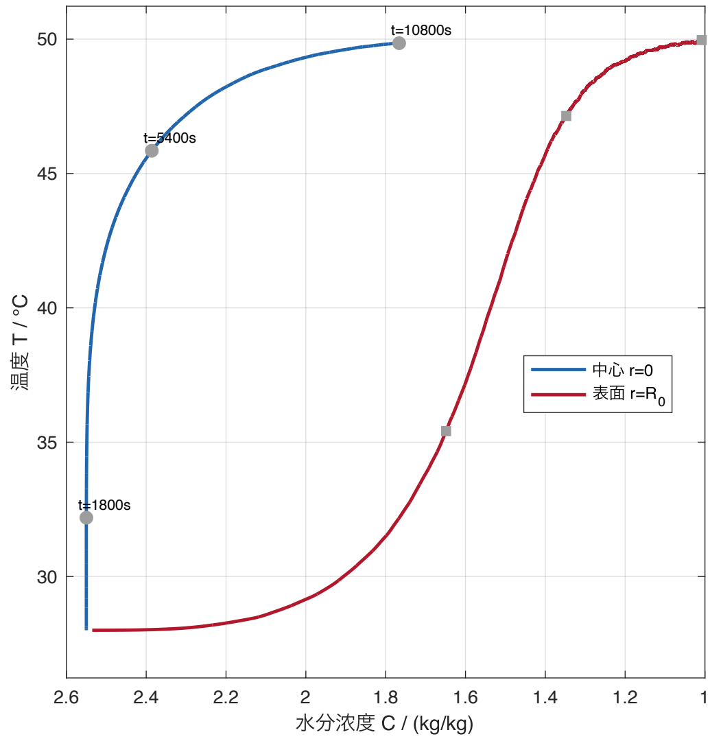
Q2 温度-水分浓度相轨迹
