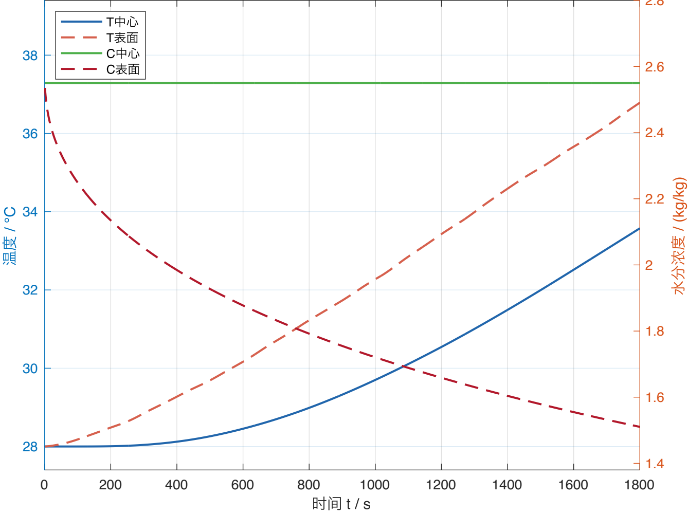
Q1 中心与表面温度、水分浓度时程曲线
