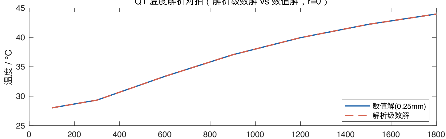
Q1 温度解析对拍 ( 解析级数解 vs 数值解, r=0 )
