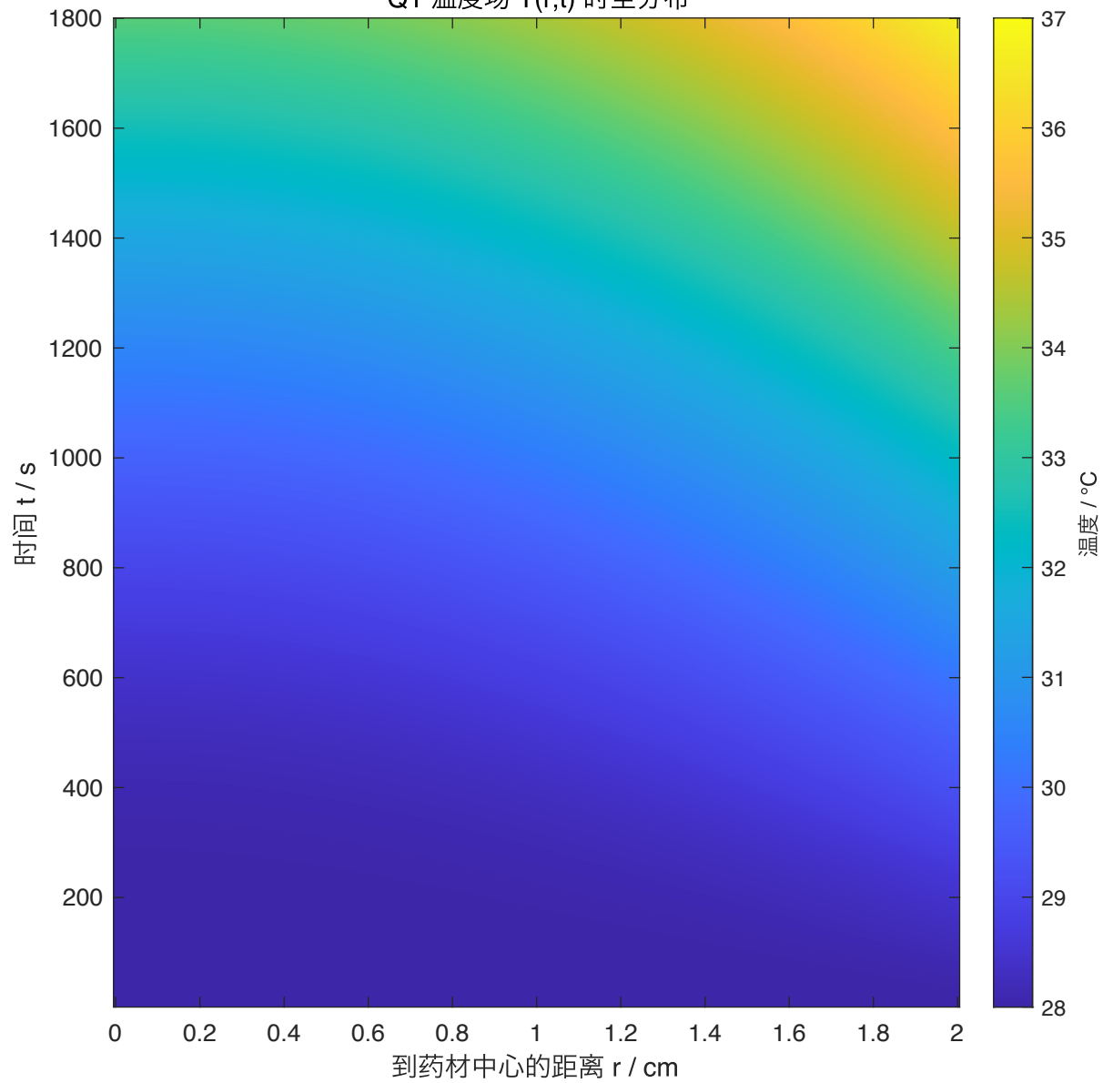
Q1 温度场 T(r,t) 时空分布
