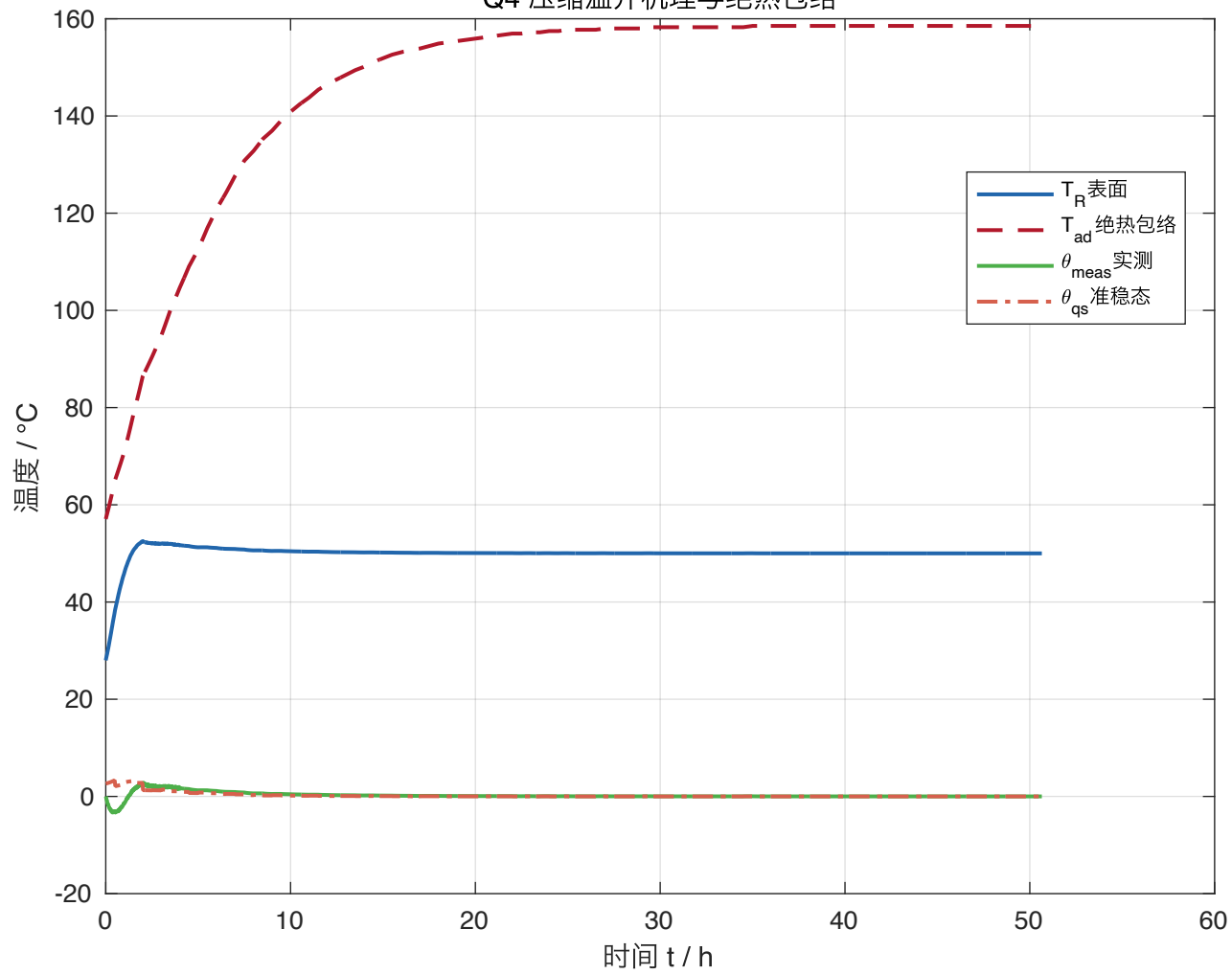
Q4 压缩温升机理与绝热包络
