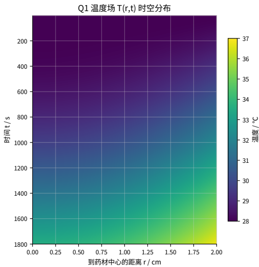
图 5-3 问题一温度场时空分布
