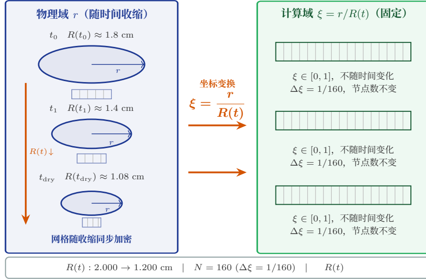
图 5-10 物质坐标变换示意图
