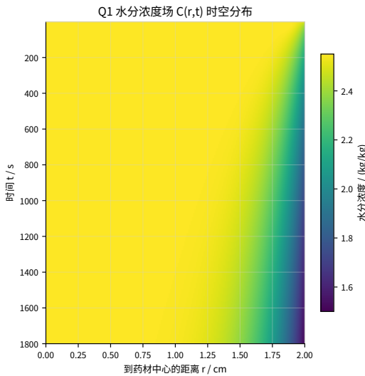
图 5-4 问题一水分浓度场时空分布
