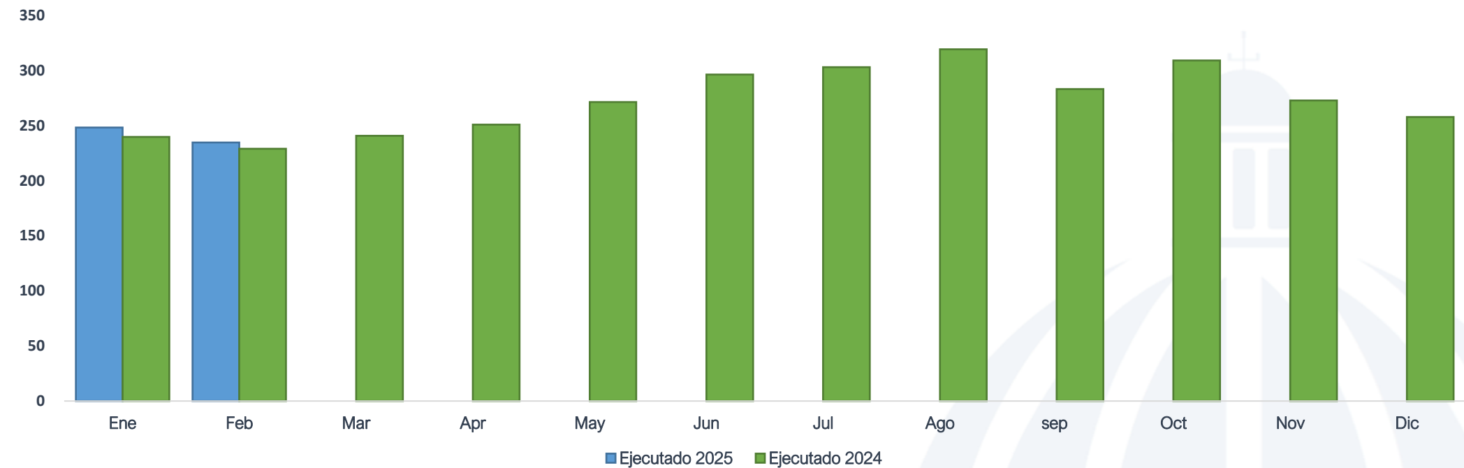
Energía Facturada Edeeste enero-febrero 2025- enero-febrero 2024 (GWh)
