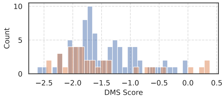
VG08 BPP22
