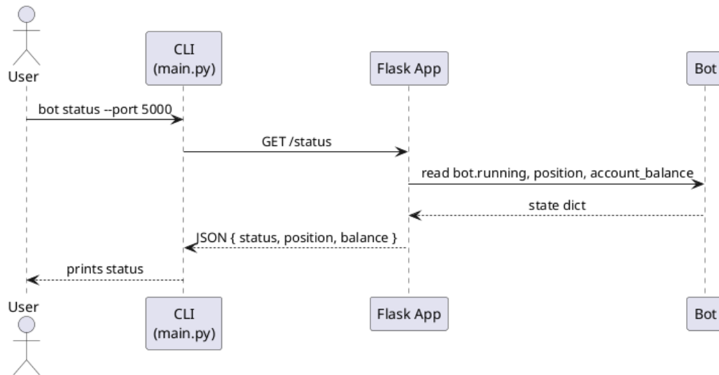
FIGURA 3.6. Diagrama del proceso de monitoreo del bot de trading.
