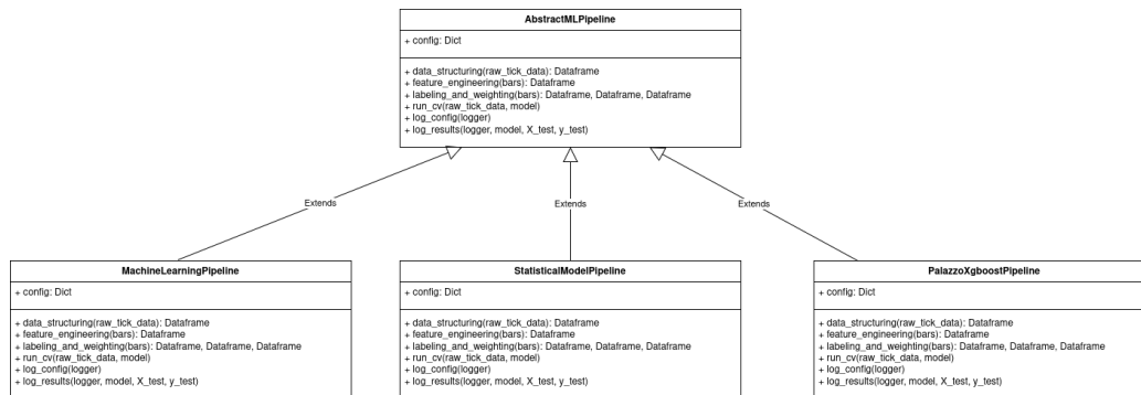
FIGURA 3.9. Estructura jerárquica de herencia de clase para AbstractMLPipeline.
