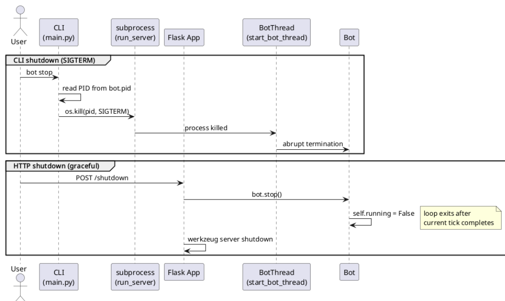
FIGURA 3.7. Diagrama del proceso de apagado del bot de trading.
