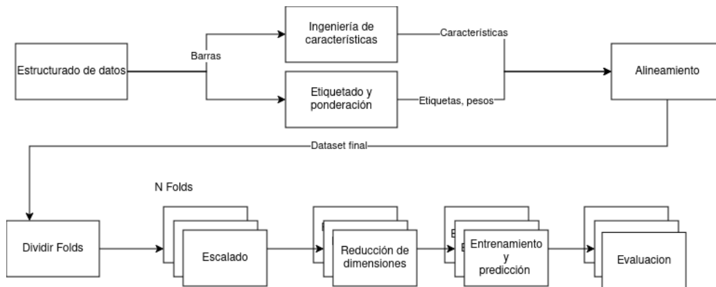
FIGURA 3.8. Flujo de datos en distintas etapas de procesamiento del pipeline.
