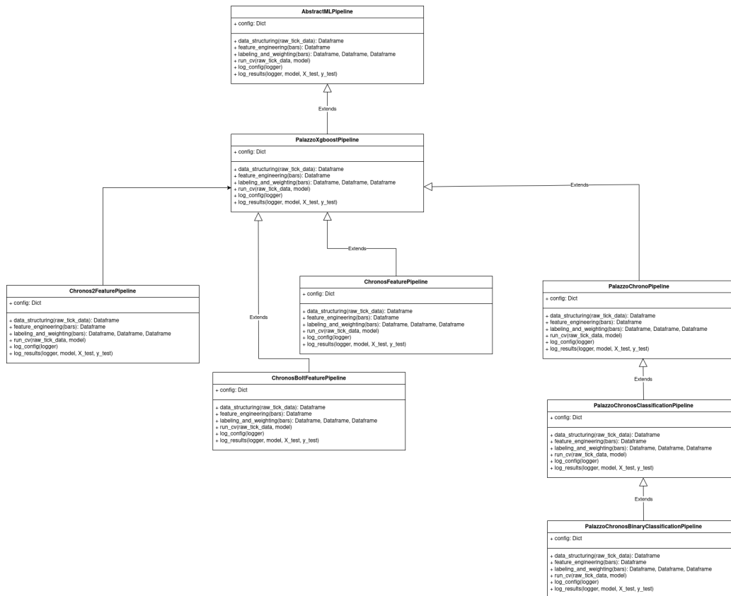
FIGURA 3.10. Estructura jerárquica de herencia de clase para los experimentos realizados con Chronos.
