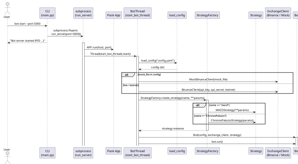
FIGURA 3.4. Diagrama del proceso de inicialización del bot.
