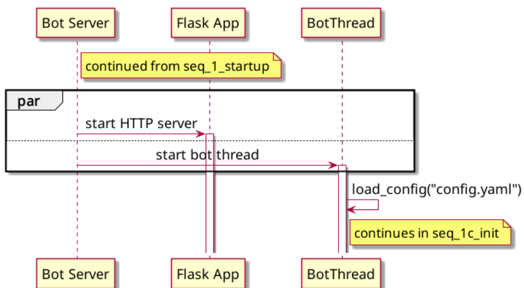
FIGURA 3.5. Diagrama del proceso de inicialización del bot - parte 2.
