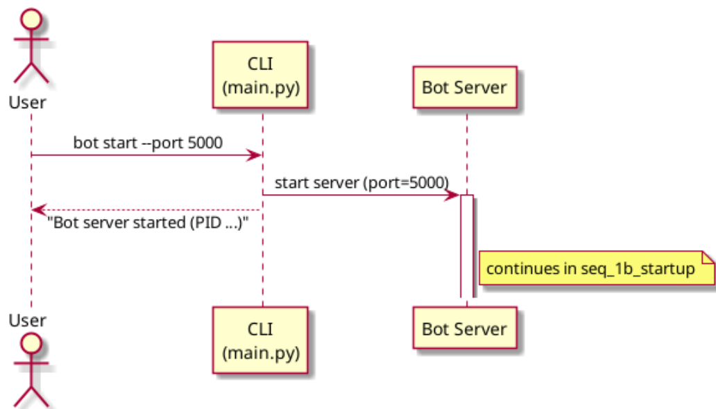
FIGURA 3.4. Diagrama del proceso de inicialización del bot - parte 1.
