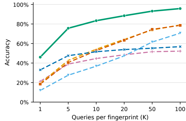
Gemma-4-12B-it
