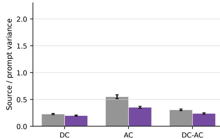
Qwen3-32B
