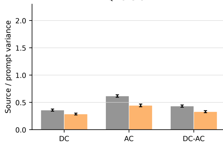
Qwen3-8B
