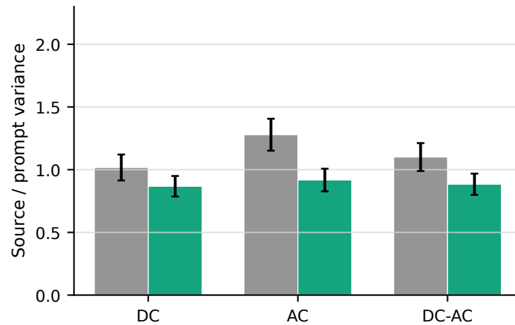
Qwen3-8B
