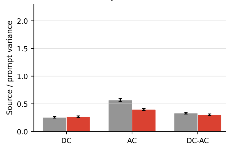
Qwen3-32B
