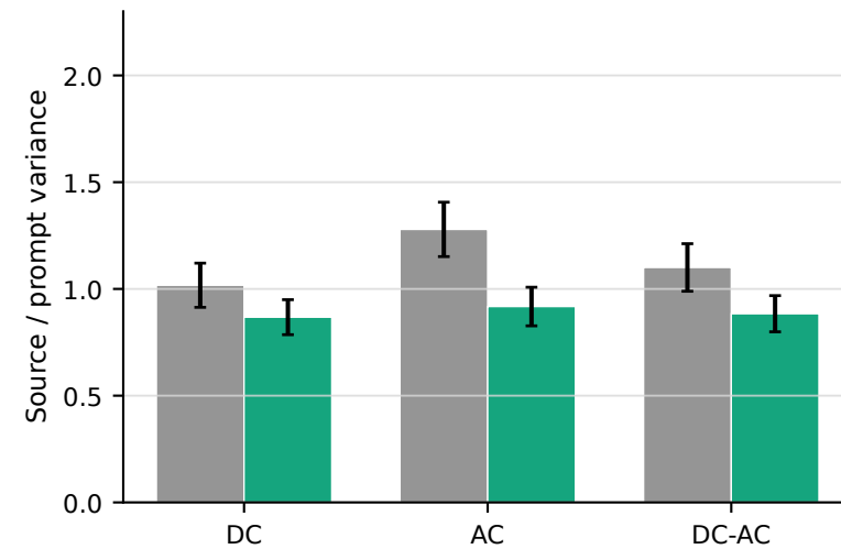
Gemma-4-12B-it
