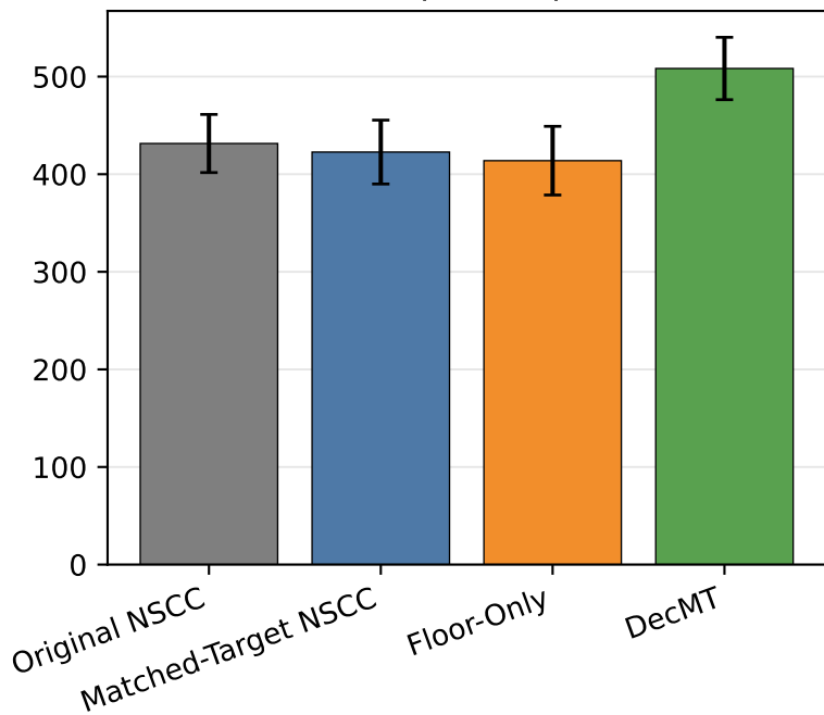
Goodput (Gbps)
