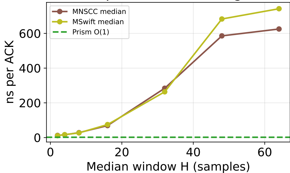
Compute scales O(H \log H)
