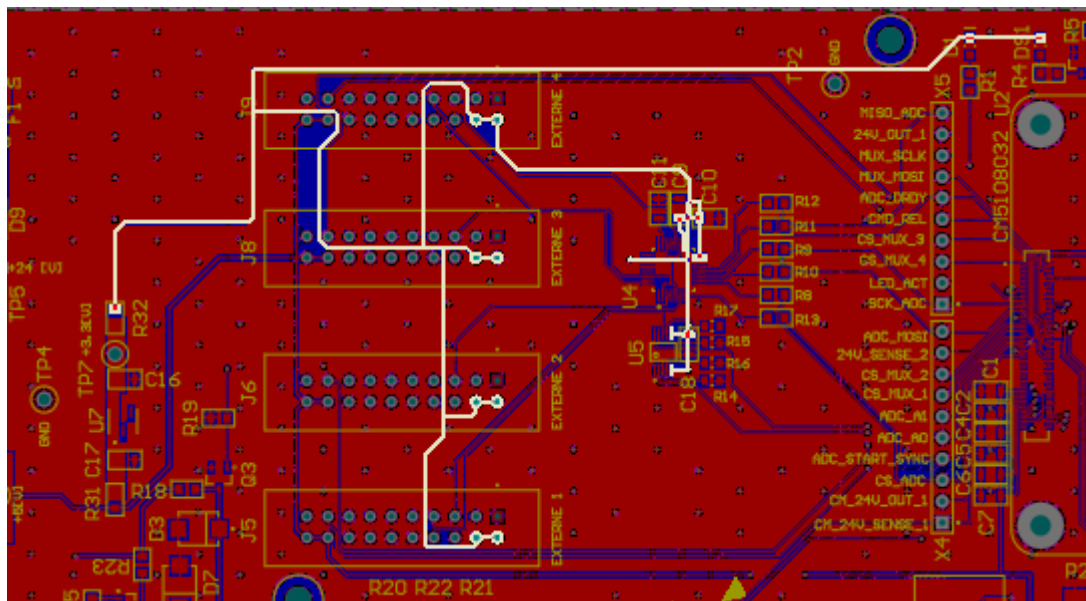
Figure 40 - Routing des pistes : Carte mère (Alimentations 3V3)
