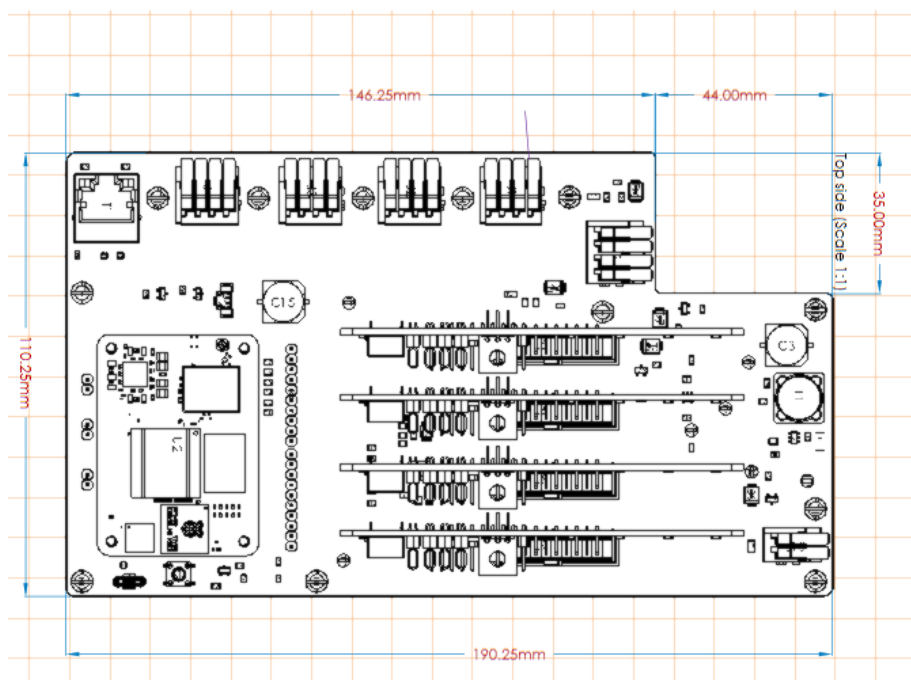
Figure 31 - PCB mère
