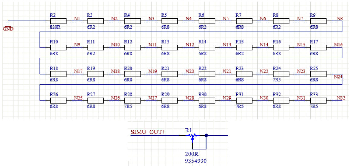
Figure 25 - Réseau de résistances simulant les sondes
