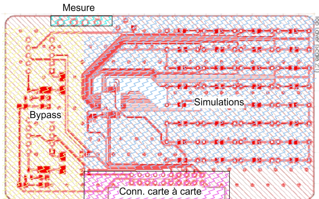
Figure 33 - Placement des composants : Carte fille
