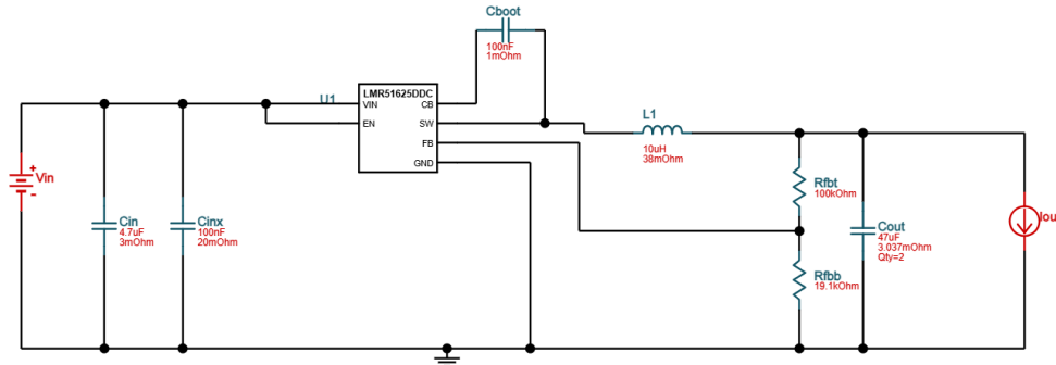
Figure 3 – Valeur calculée par le calculateur 1
