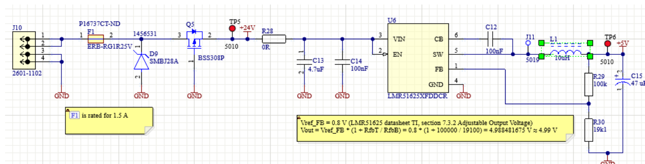
Figure 2 - Bloc d'alimentation stepdown, protections à l'entrée
