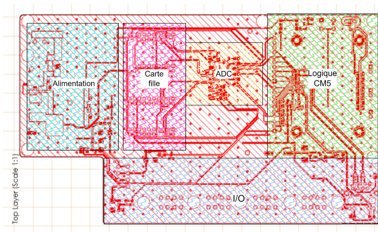
Figure 34 - Placement des composants : Carte mère
