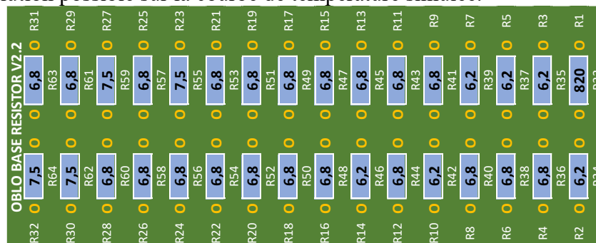
Figure 26 Implantation du réseau de résistances sur la carte fille actuelle d'oblo
