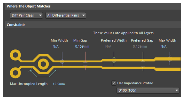
Figure 44 - Paramétrage règles lignes différentielles (impédance)
