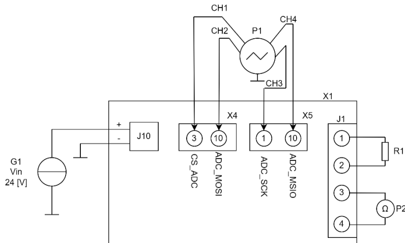
Figure 67 - Schéma de mesure : Mesure communication SPI ADC
