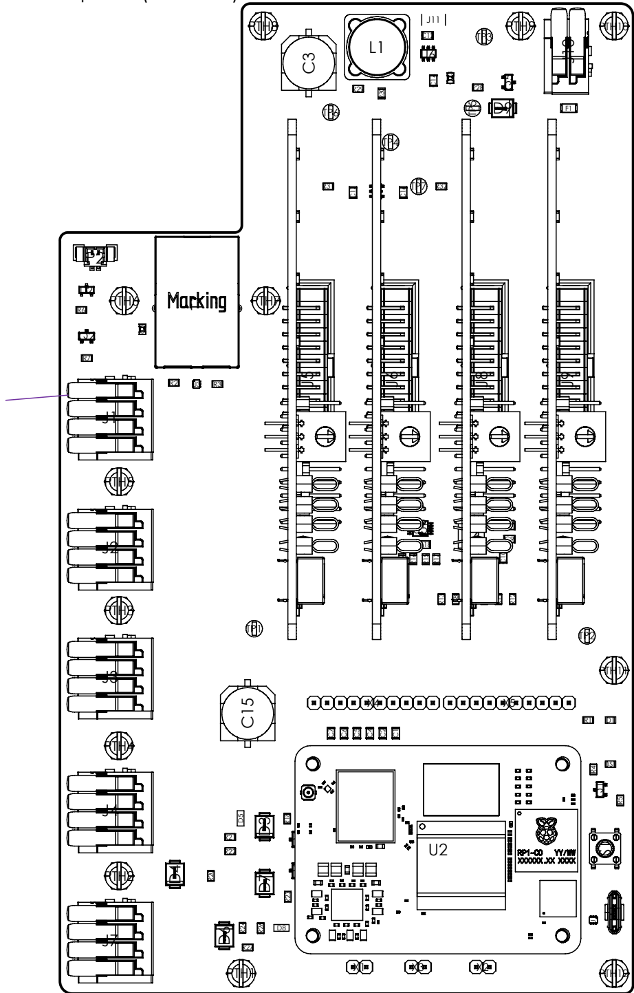
Top side (Scale 1:1)
