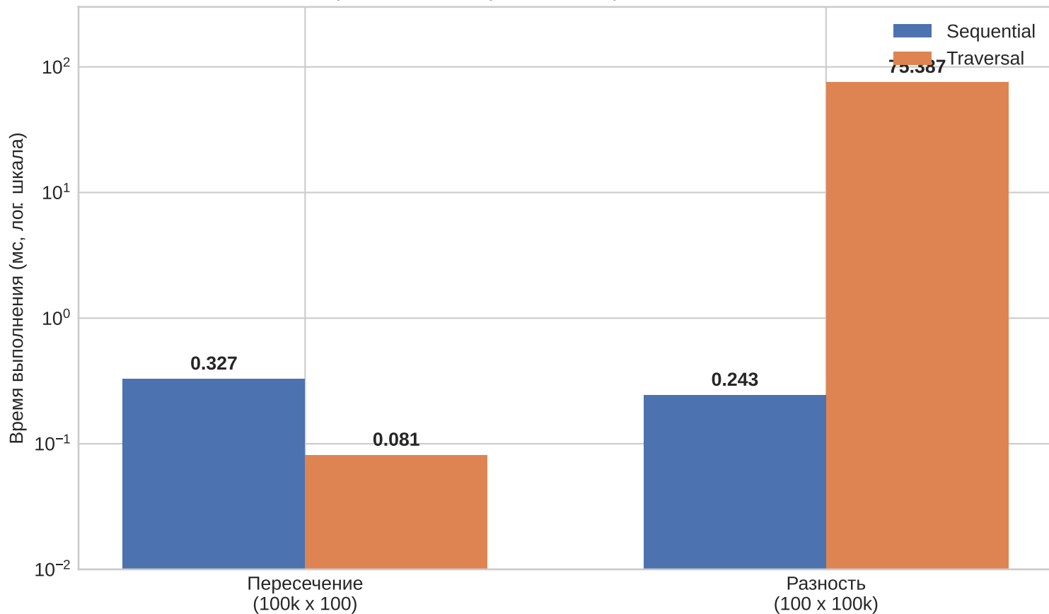
Сравнение алгоритмов: Sequential vs Traversal
