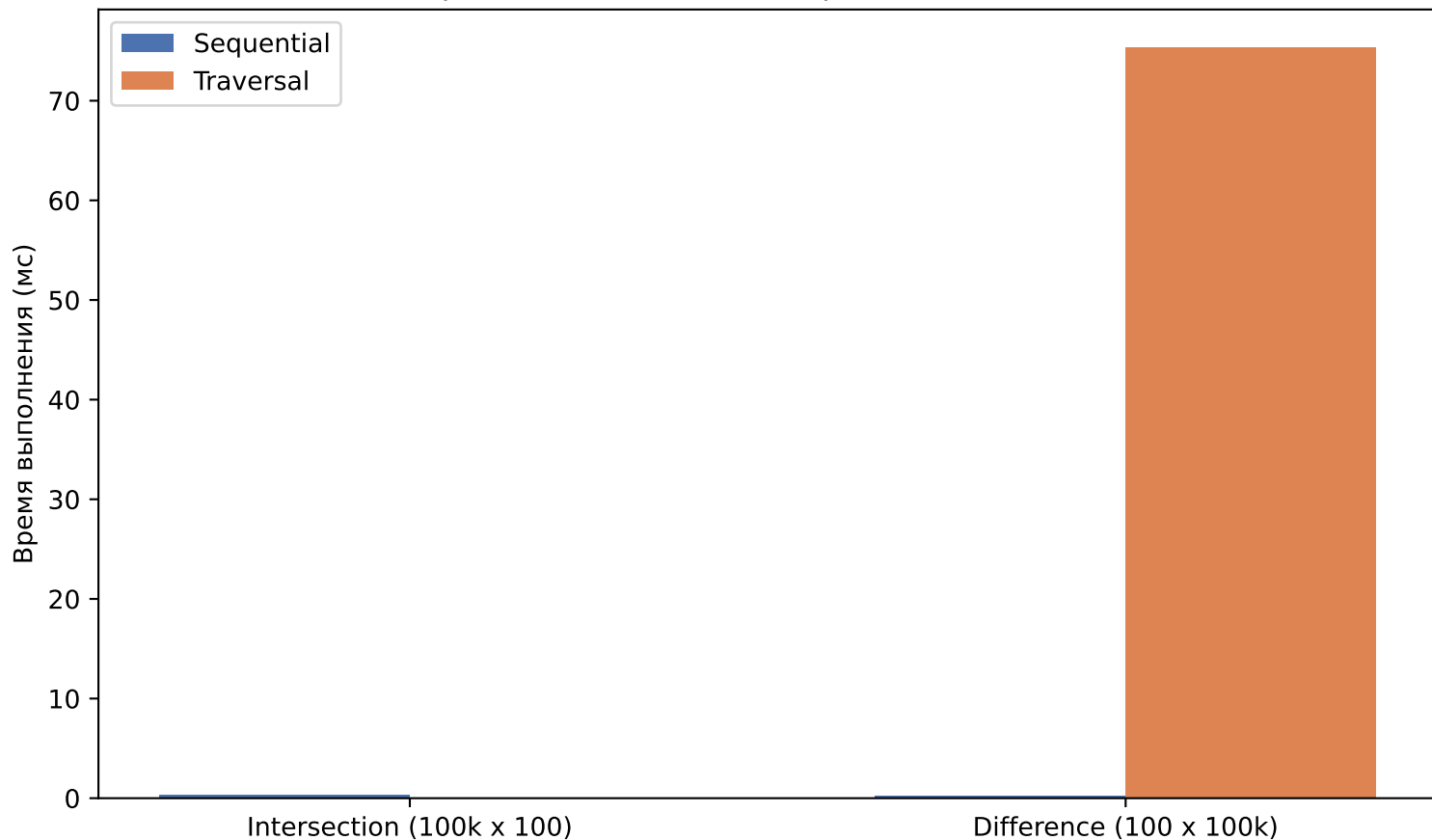
Сравнение подходов Sequential и Traversal
