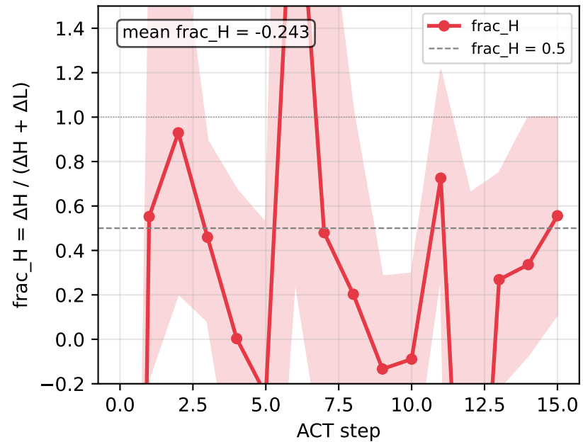
H-update share (sudoku)
