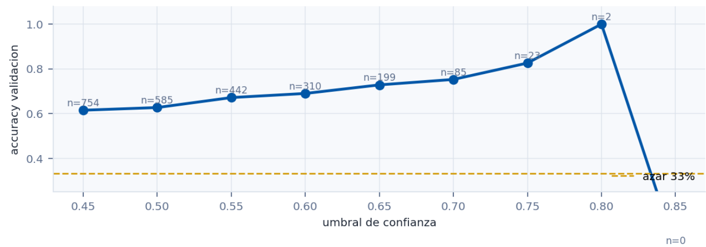
Accuracy por umbral de confianza en validacion
