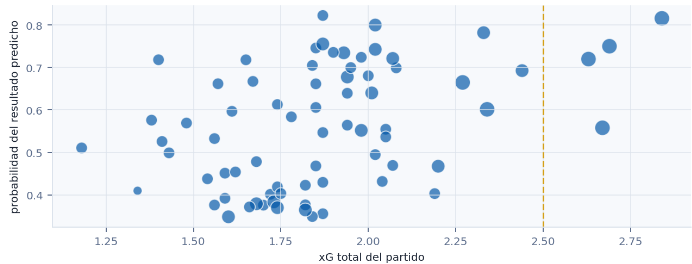
Cada punto es un partido de fase de grupos. Puntos mas grandes indican marcadores recomendados con mayor total de goles.
