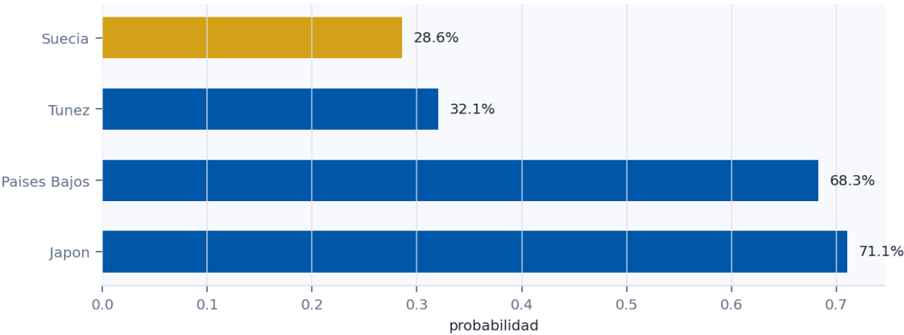
Grupo F: probabilidad de clasificar directo
