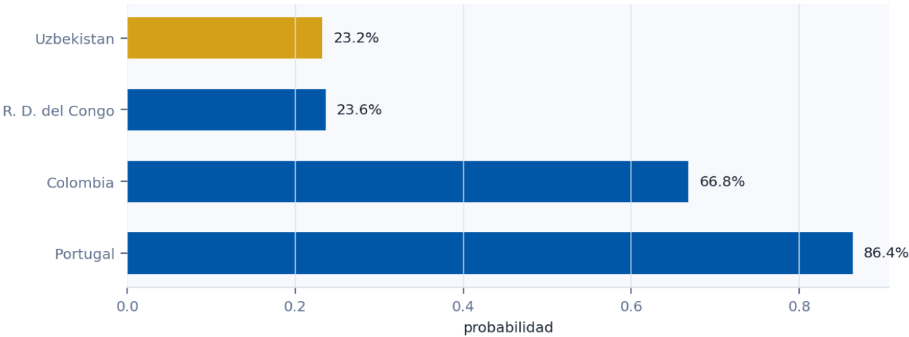
Grupo K: probabilidad de clasificar directo
