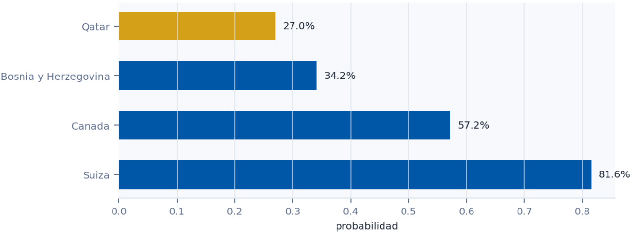
Grupo B: probabilidad de clasificar directo
