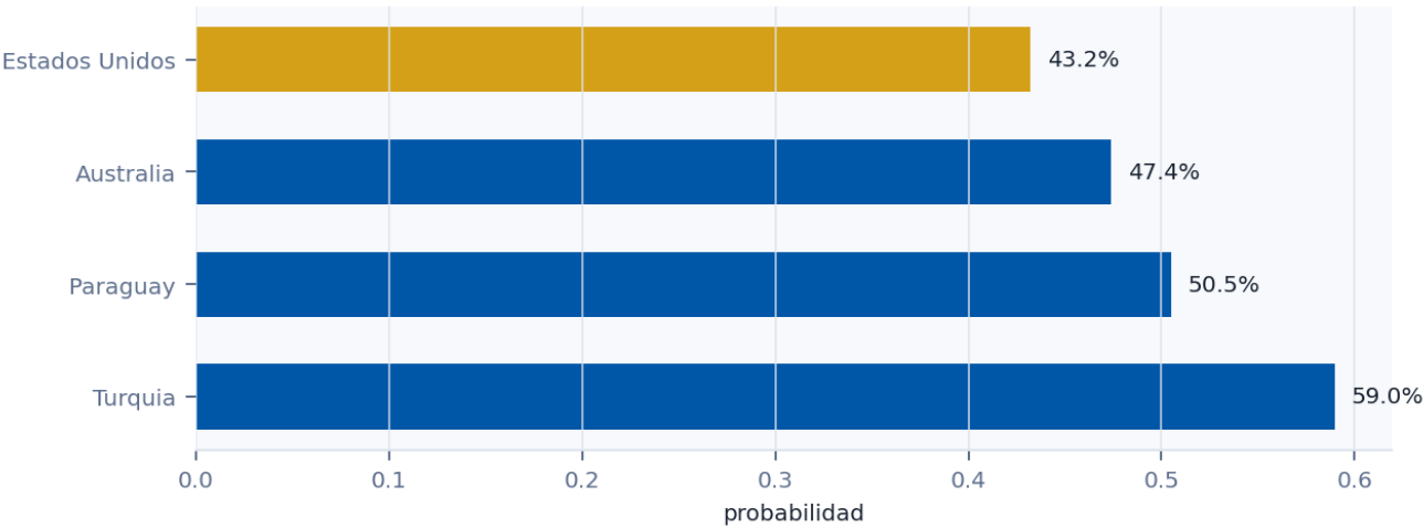
Grupo D: probabilidad de clasificar directo
