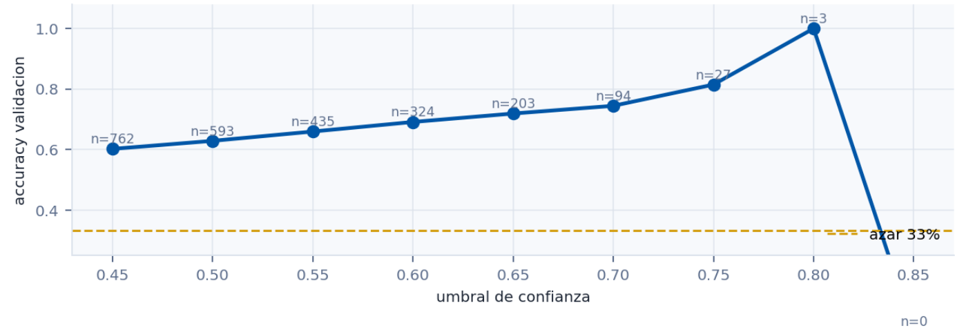
Accuracy por umbral de confianza en validacion
