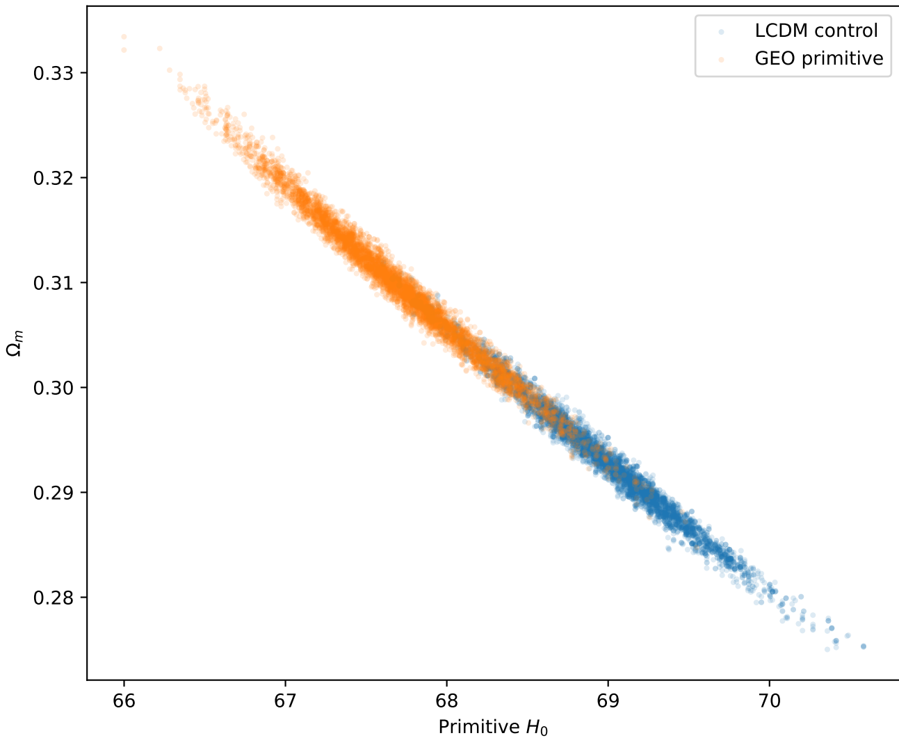
H_0 -- \Omega_m posterior structure
