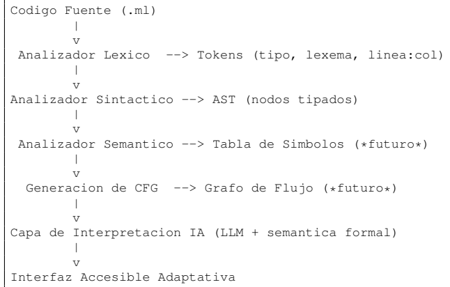
Fig. 1. Pipeline del Compilador Aumentado con IA. Las fases marcadas como “futuro” están planificadas pero aún no implementadas.
