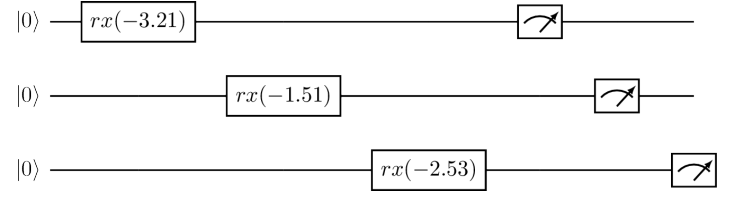
(b) RxRxToRx Output
