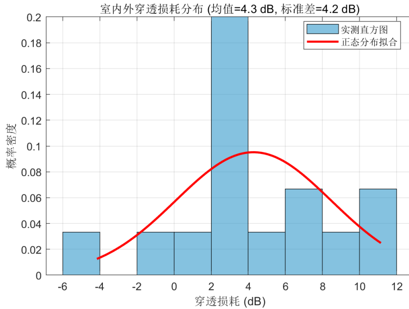
图 3: 建筑物穿透损耗分布
