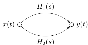
图 5.12: 并联
