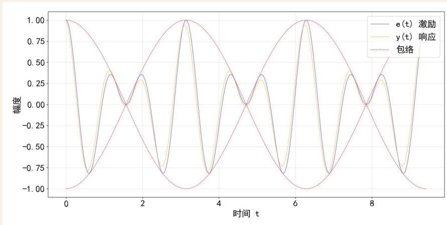
图 5.5: 调幅信号通过具有负群时延系统的响应
