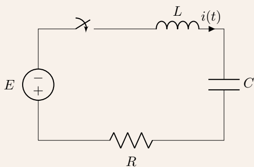
(a) 时域电路
