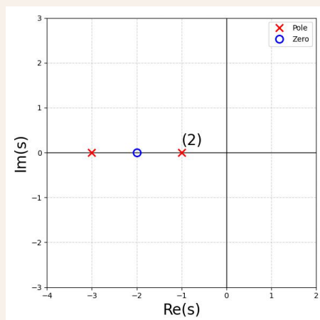
图 5.7: 零极点图(1)
