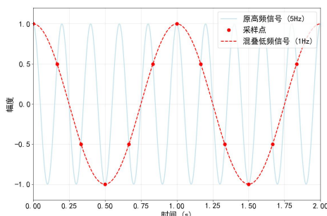
图 4.2: 正弦波的混叠现象
