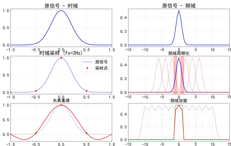
图 4.3: 混叠的频域分析
