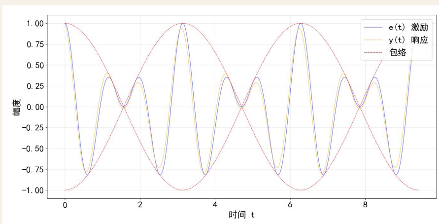
图 5.12: 调幅信号通过具有负群时延系统的响应
