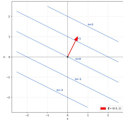
图 4.7: 二维空间中 e^{2\pi i \mathbf{x} \cdot \boldsymbol{\xi}} 的等相面示意图
