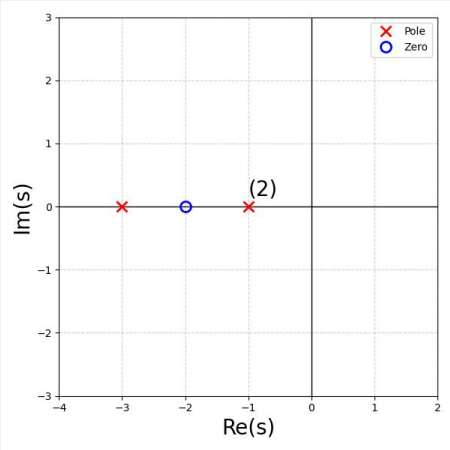
图 5.5: 零极点图(1)
