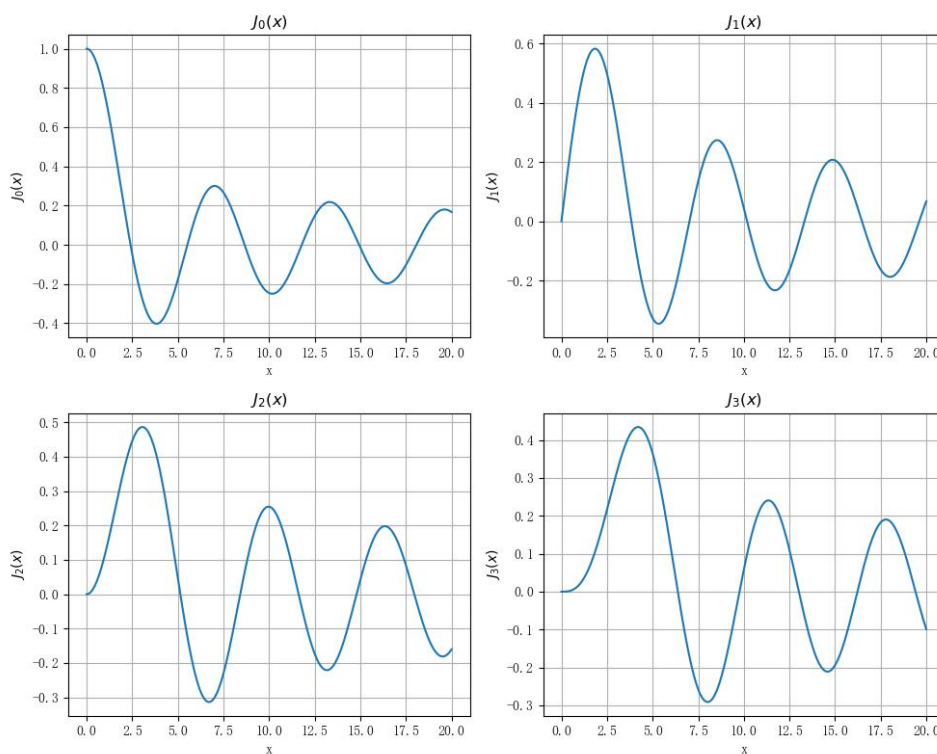
图 1.4: 第一类贝塞尔函数 J_n(x) , n = 0, 1, 2, 3 的图像
