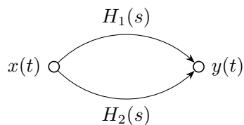
图 5.10: 并联
