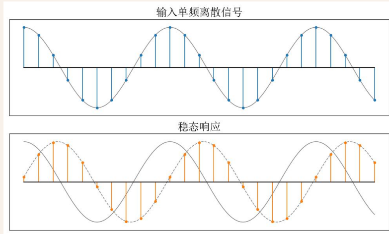
图 7.3: 离散系统的相延迟示意图
