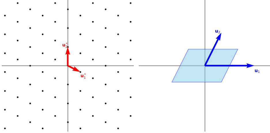
图 4.9: 格采样示意图
