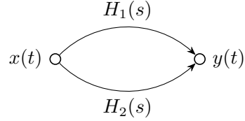
图 5.10: 并联
