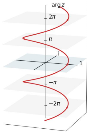
图 3.3: 相频特性解卷绕示意图
