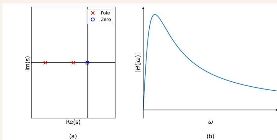
图 5.8: 零极点图与幅频特性曲线 (1)
