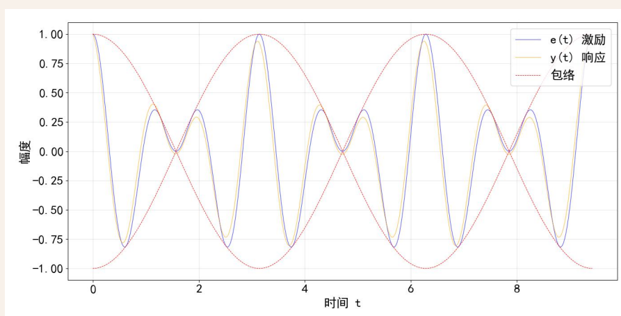
图 5.5: 调幅信号通过具有负群时延系统的响应
