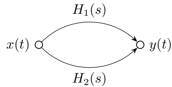
图 5.12: 并联
