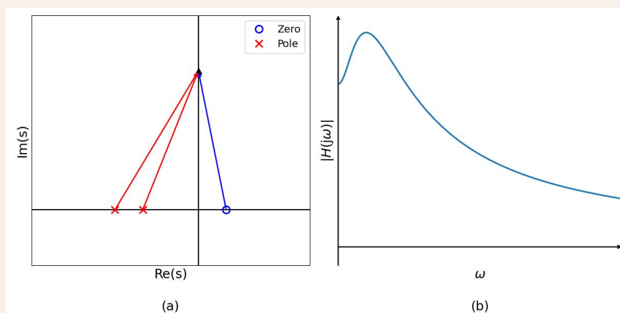
图 5.10: 零极点图与幅频特性曲线 (3)
