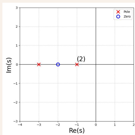
图 5.7: 零极点图 (1)
