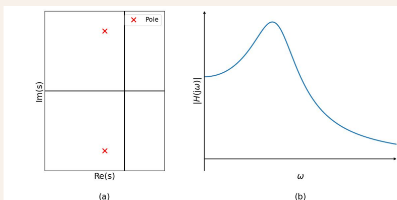
图 5.9: 零极点图与幅频特性曲线 (2)
