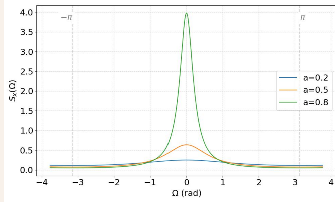
图 6.5: 指数序列的能量谱密度
