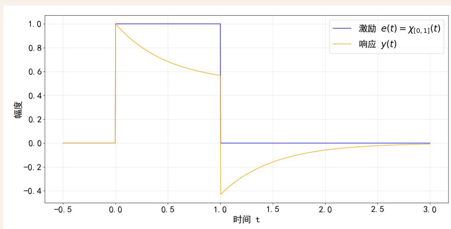
图 5.6: 暂态信号通过原系统的响应
