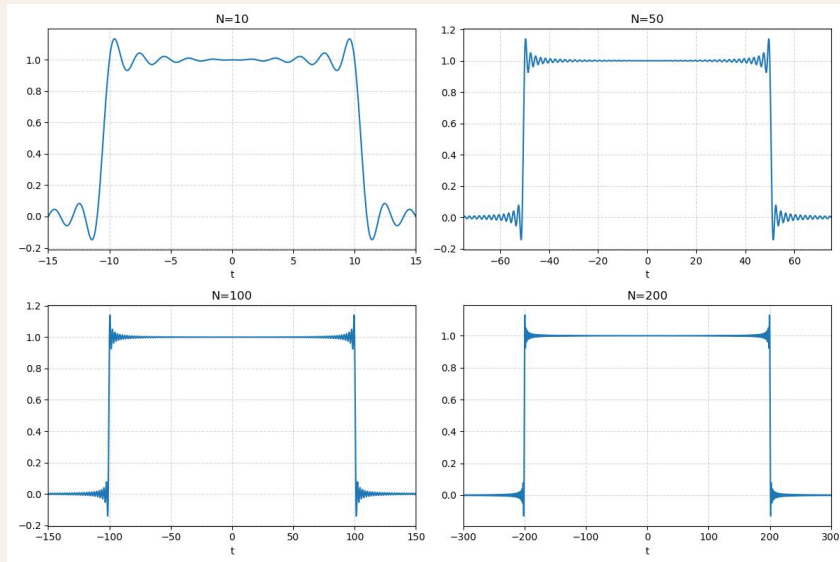
图 4.4: \text{sinc}(t) * \text{III} 的前 N 项和
