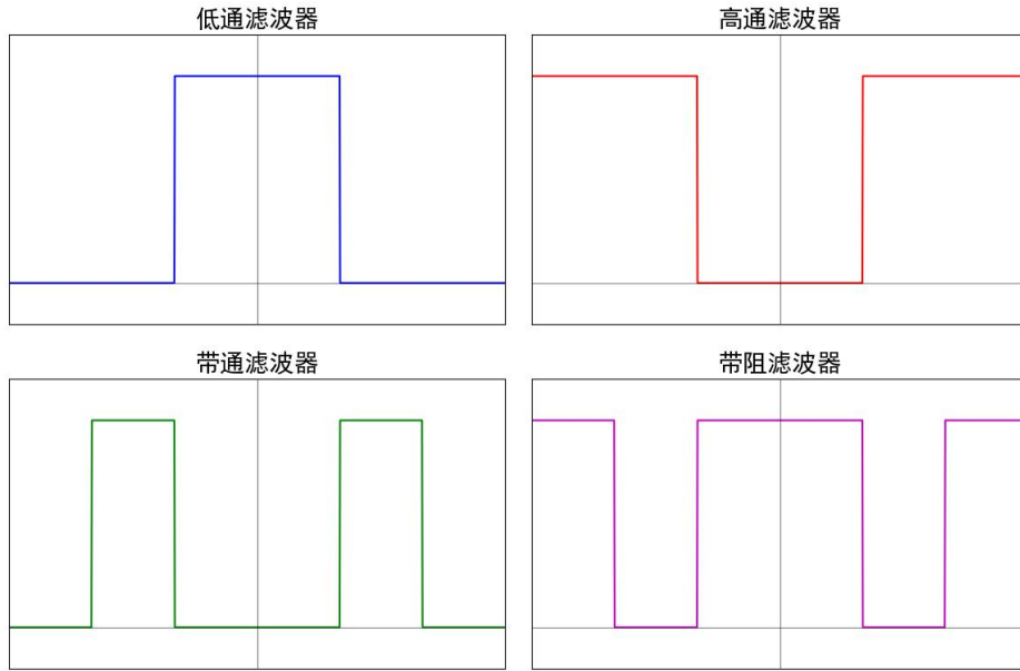
图 3.2: 理想滤波器的幅频特性
