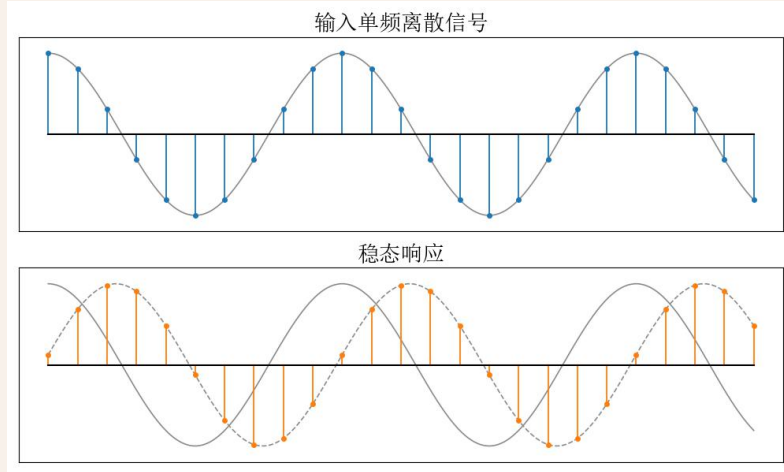
图 7.3: 离散系统的相时延示意图
