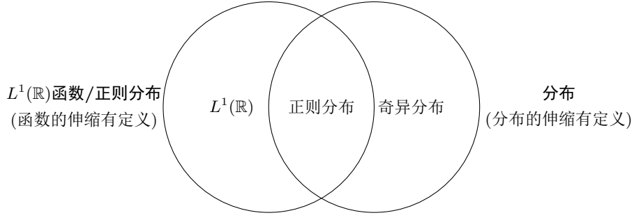
图 2.3: 伸缩的定义范围示意图
