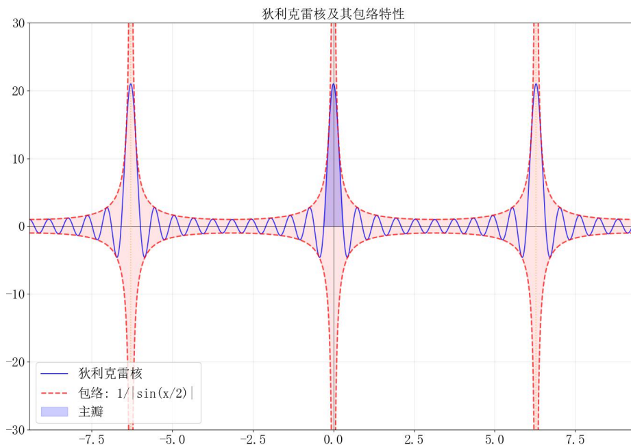
图 A.1: 狄利克雷核 D_N(t) 的函数图像
