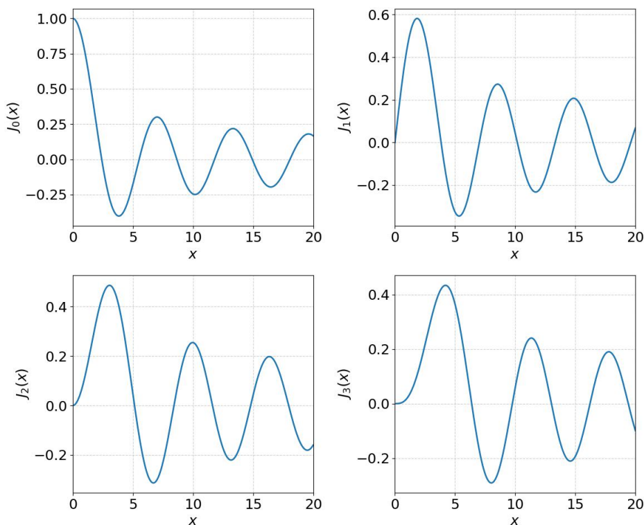
图 1.5: 第一类贝塞尔函数 J_n(x) , n = 0, 1, 2, 3 的图像
