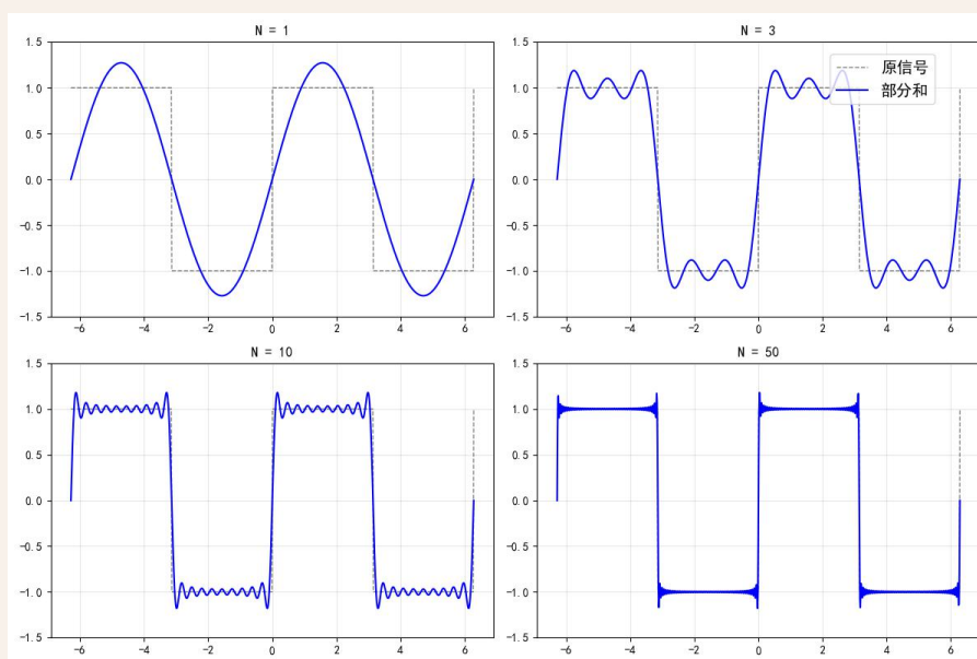
图 2.2: 吉布斯现象示意图
