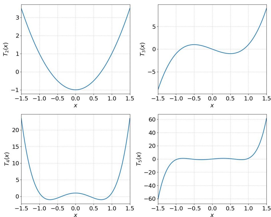
图 1.4: 第一类切比雪夫多项式 T_n(x), n = 2, 3, 4, 5 的图像
