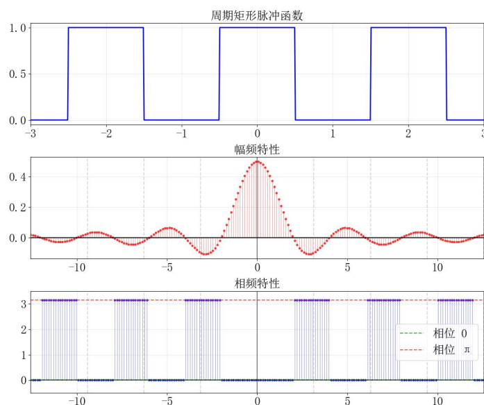
图 2.1: 周期矩形脉冲信号及其频谱
