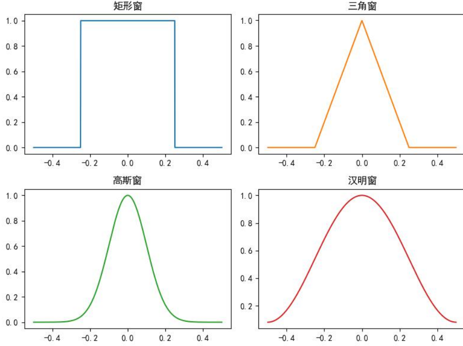
图 4.10: 常见窗函数示意图
