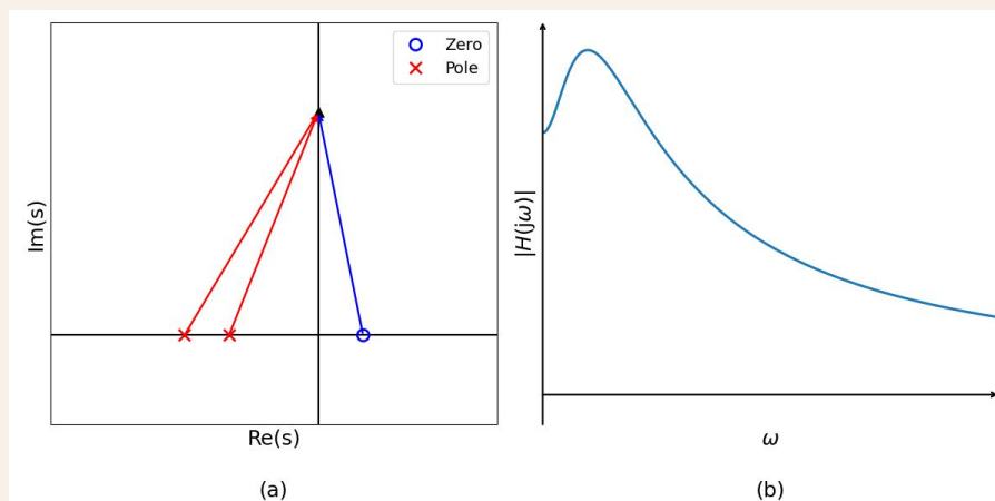
图 5.8: 零极点图与幅频特性曲线(3)
