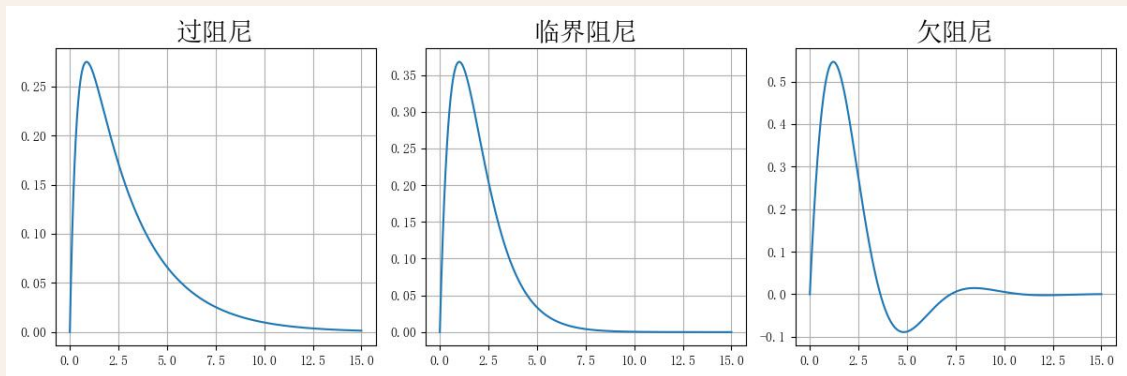
图 5.4: 不同阻尼状态下的电流响应
