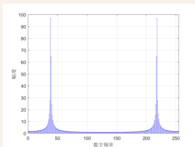
图 6.4: 256点离散傅里叶变换
