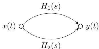
图 5.12: 并联
