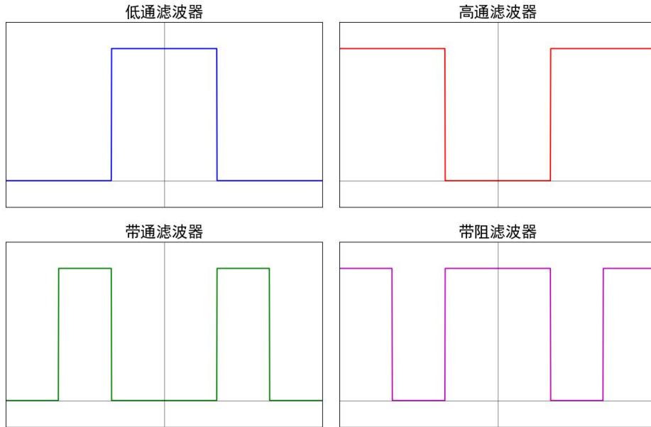
图 3.2: 理想滤波器的幅频特性
