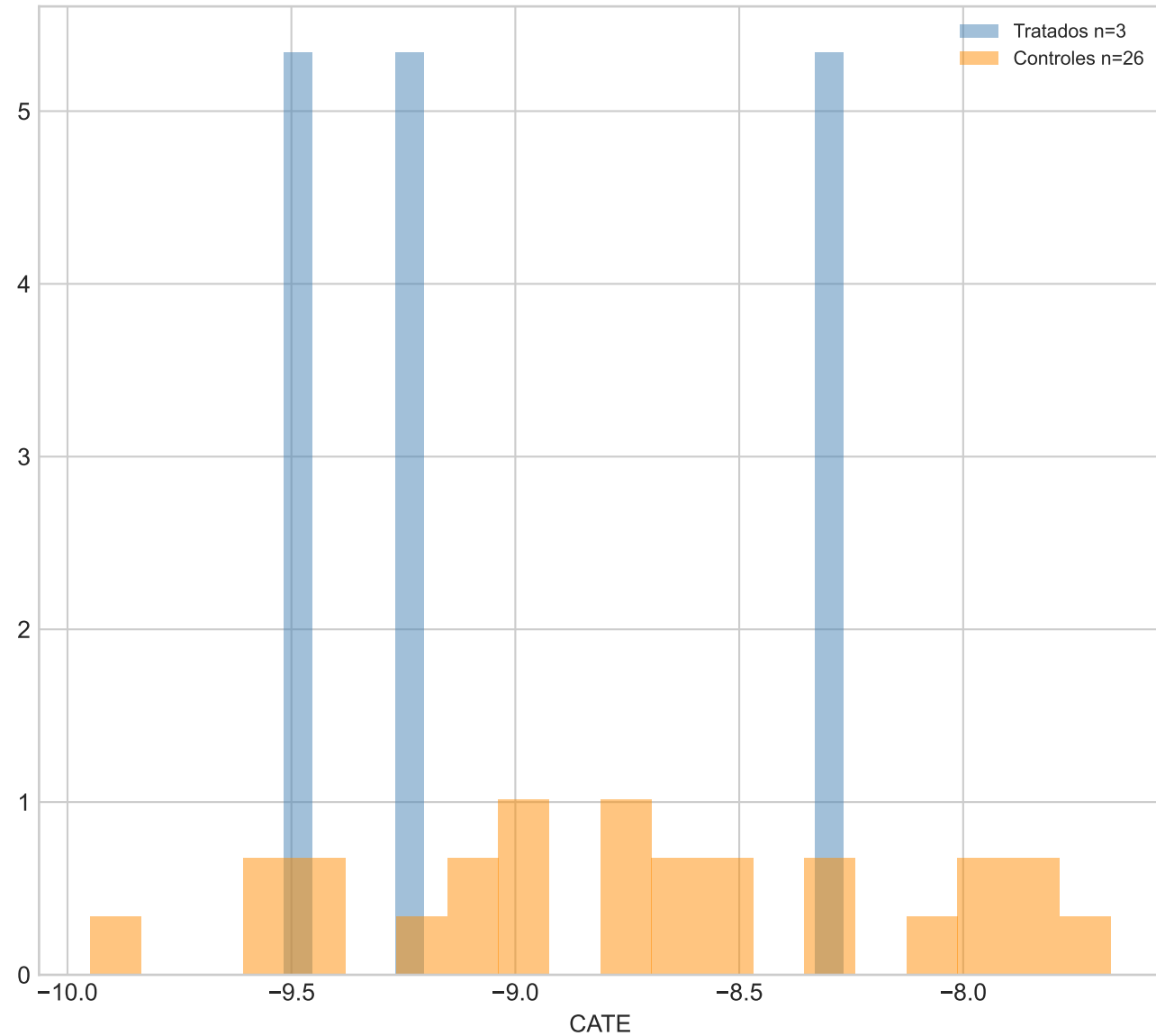
Cola baja \hat{r} \leq p_{10} = -7.67 Muestra completa (robustez)
