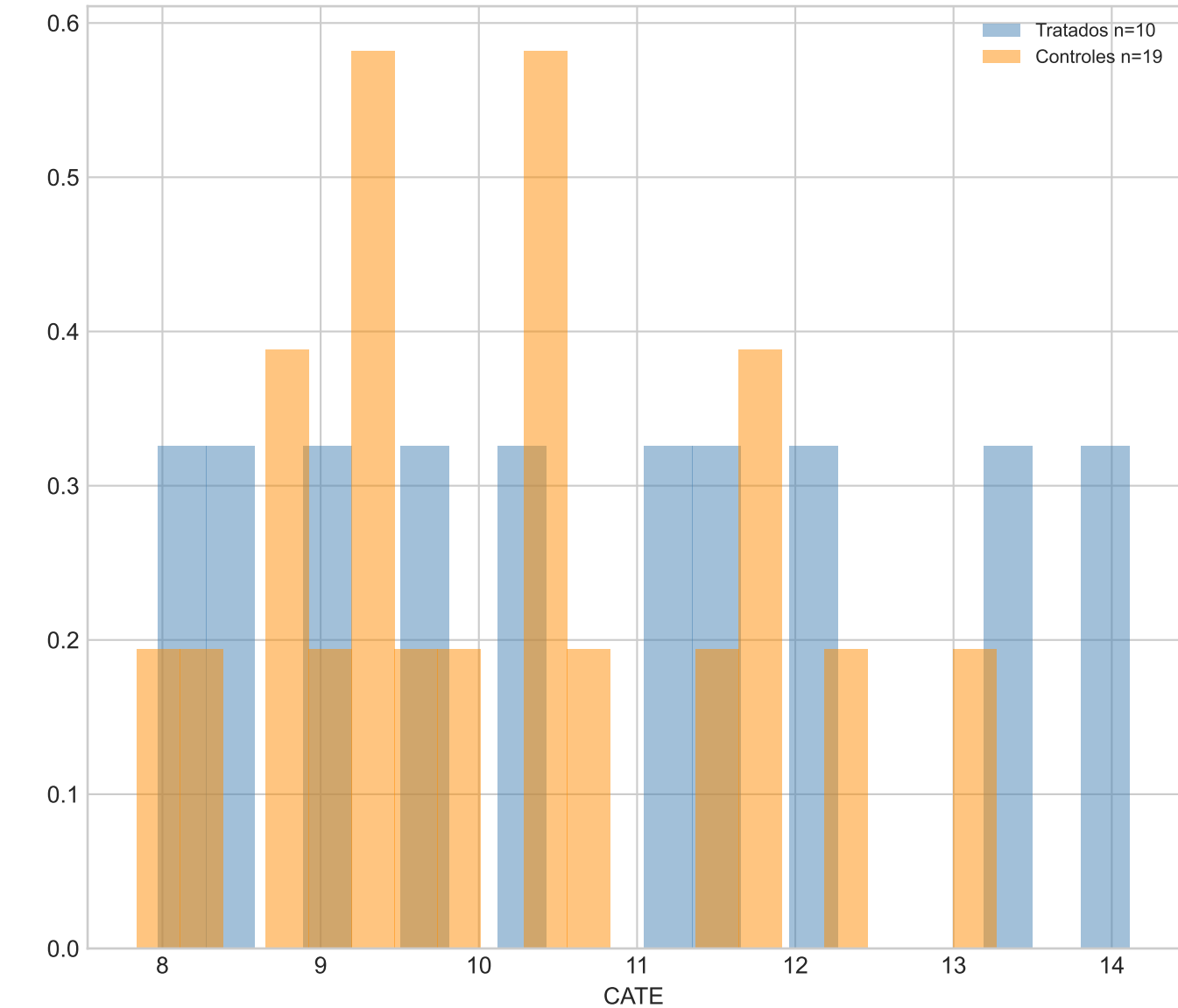
Cola alta \hat{r} \geq p_{90} = 7.84 Muestra completa (robustez)
