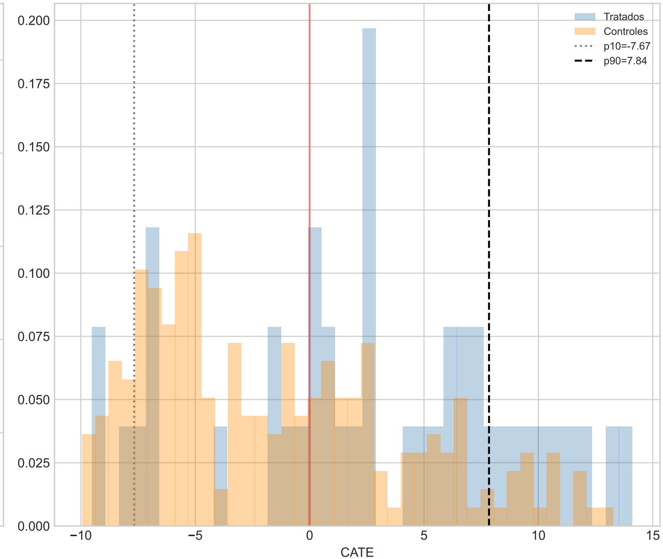
Distribución completa CATE Muestra completa (robustez)
