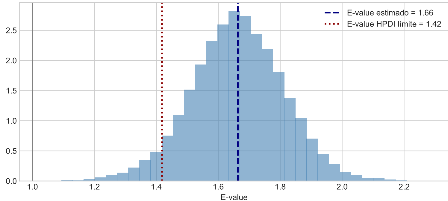
E-value posterior — Muestra completa (robustez)
